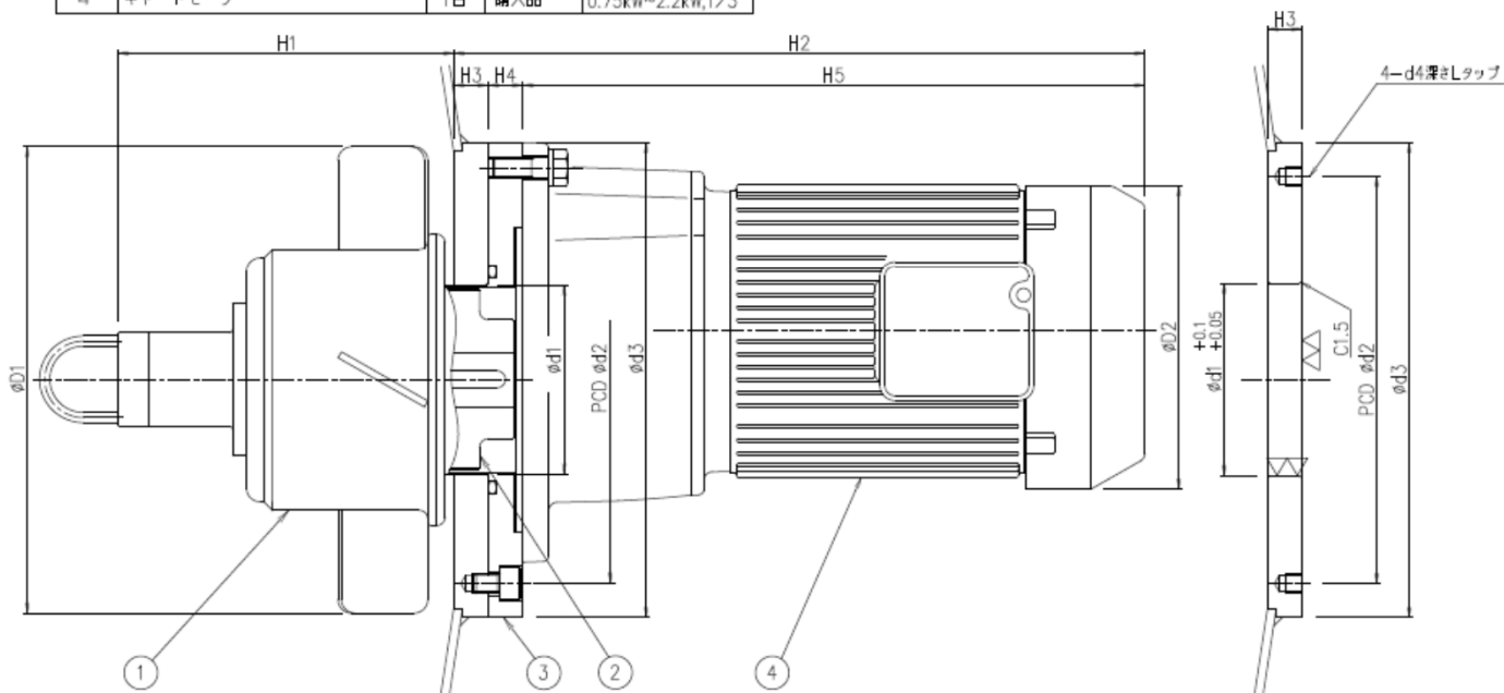
容器取付部寸法図
